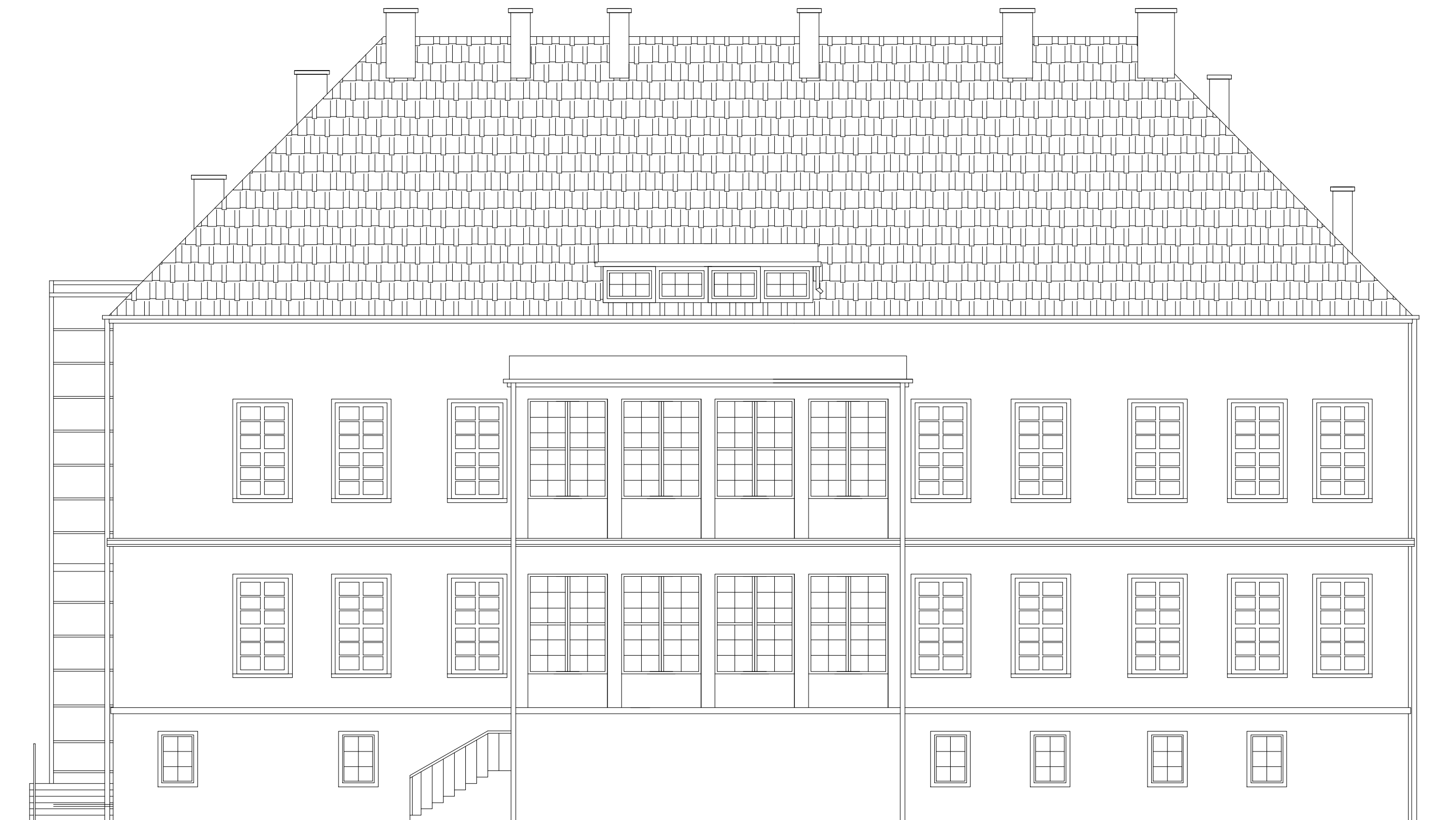
ELEWACJA ZACHODNIA
